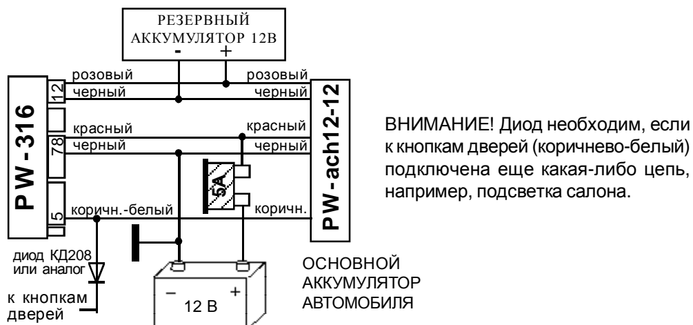
Рис.3. Подключение резервного аккумулятора и контроллера заряда PW-ach12-12.
