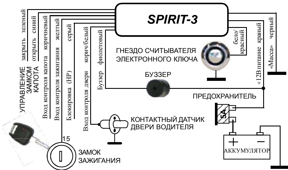
Рис. 1. Схема подключения.
